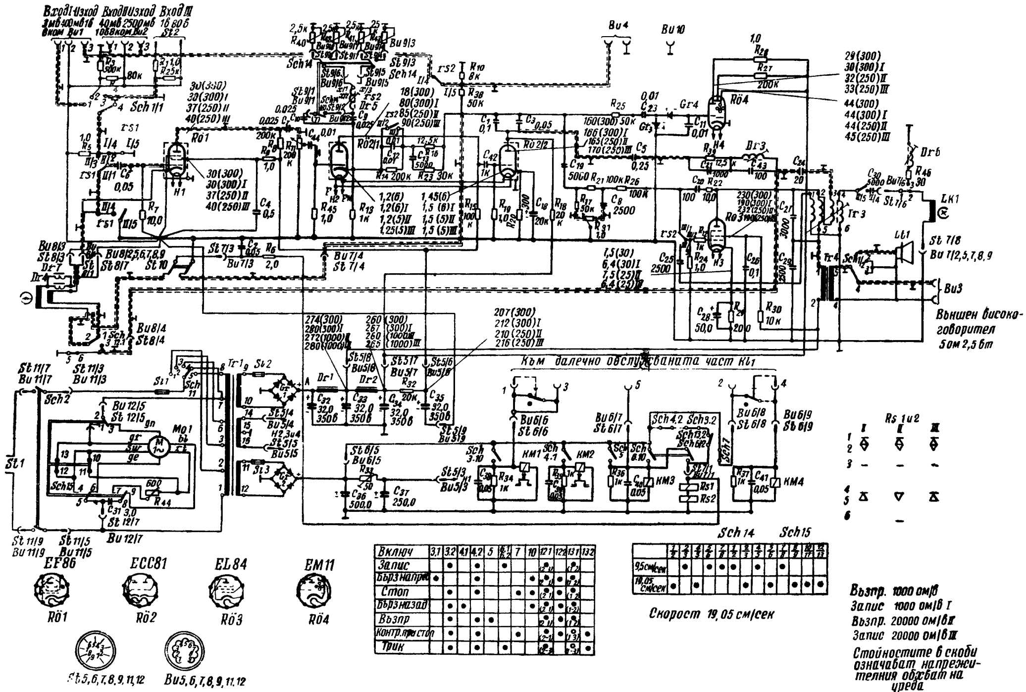
Фиг. 64. Схема на магнитофон „Смарагд“
