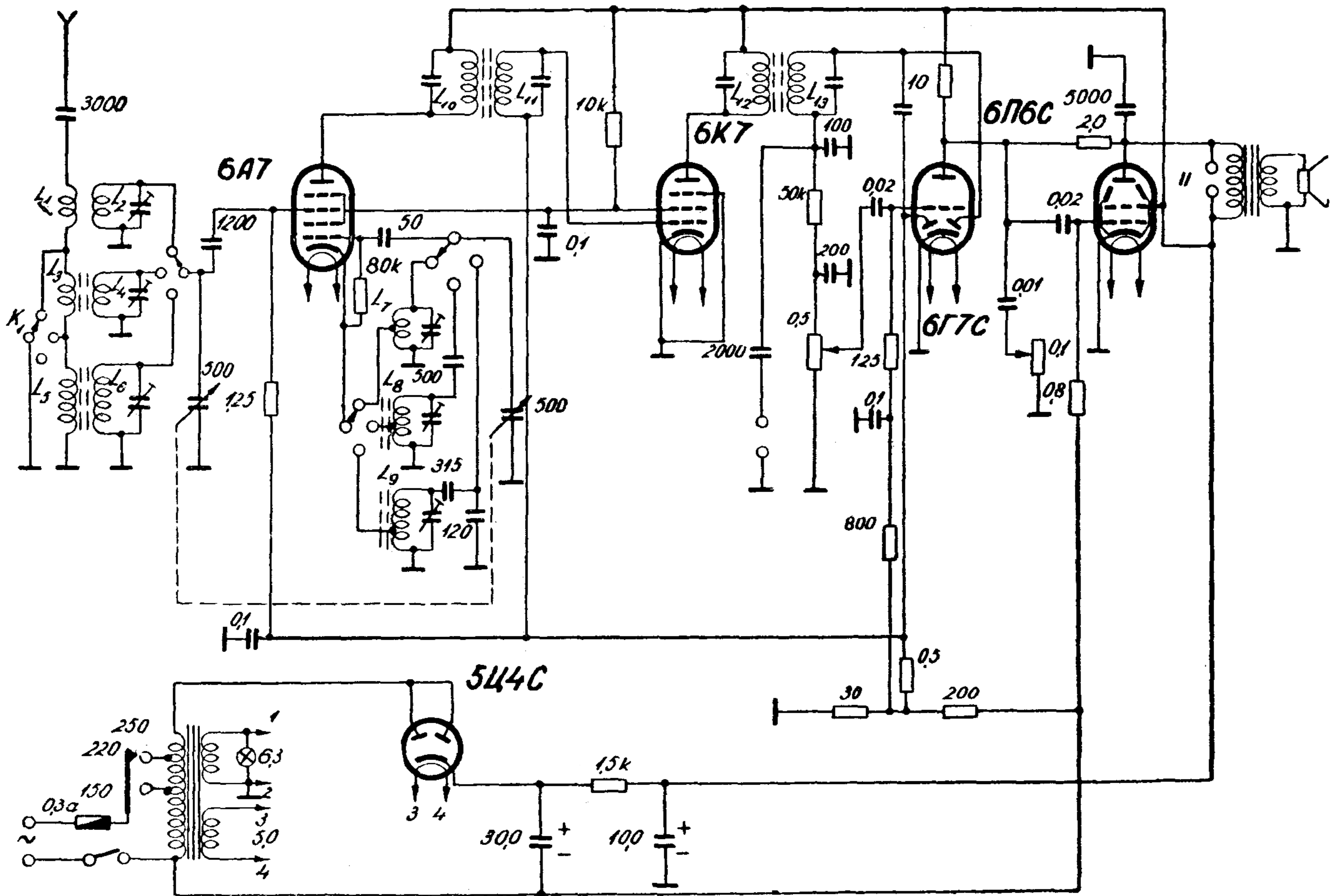
Обхват: КВ 16 ÷ 50 м (18,7 ÷ 6 мГц), СВ 197 ÷ 575 м (1520 ÷ 520 кГц), ДВ 750 ÷ 200 м (400 ÷ 250 кГц). МЧ = 468 кГц
