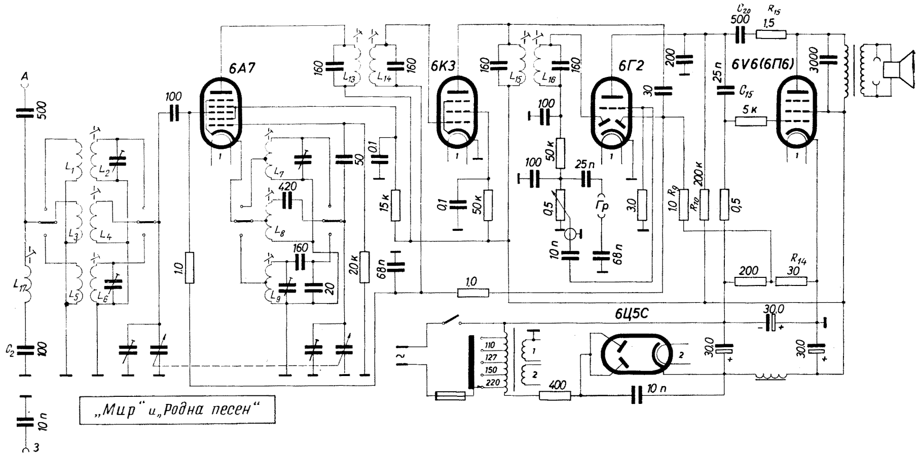
Фиг. 2.4.6. Схема на радиоприемниците „Мир“ и „Родна песен“ със съветски лампи
