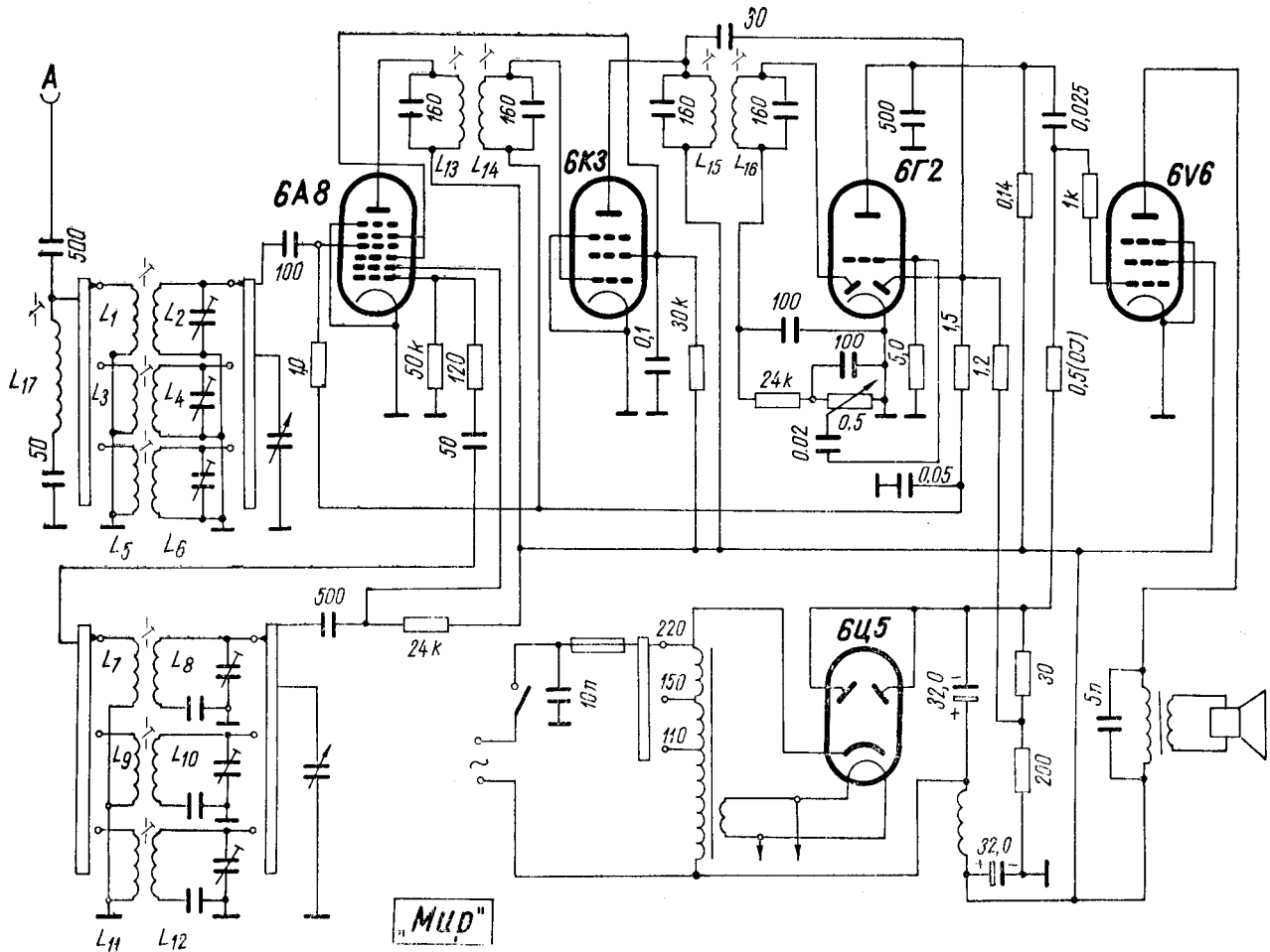
Фиг. 2.4.9. Схема на радиоприемника „Мир“ със съветски лампи
