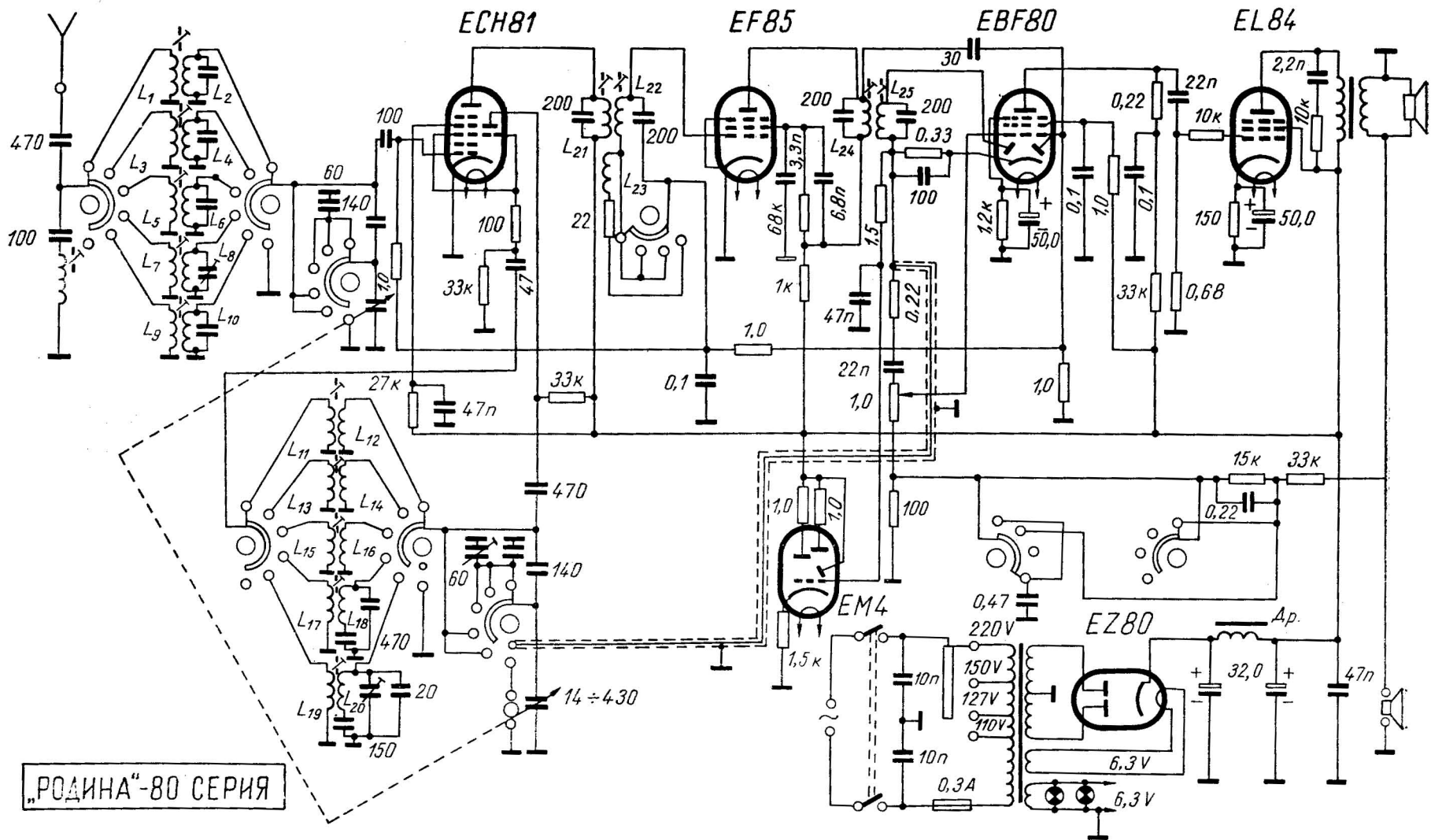
Фиг. 2.9.6. Схема на радиоприемника „Родина“ с лампи серия E80
