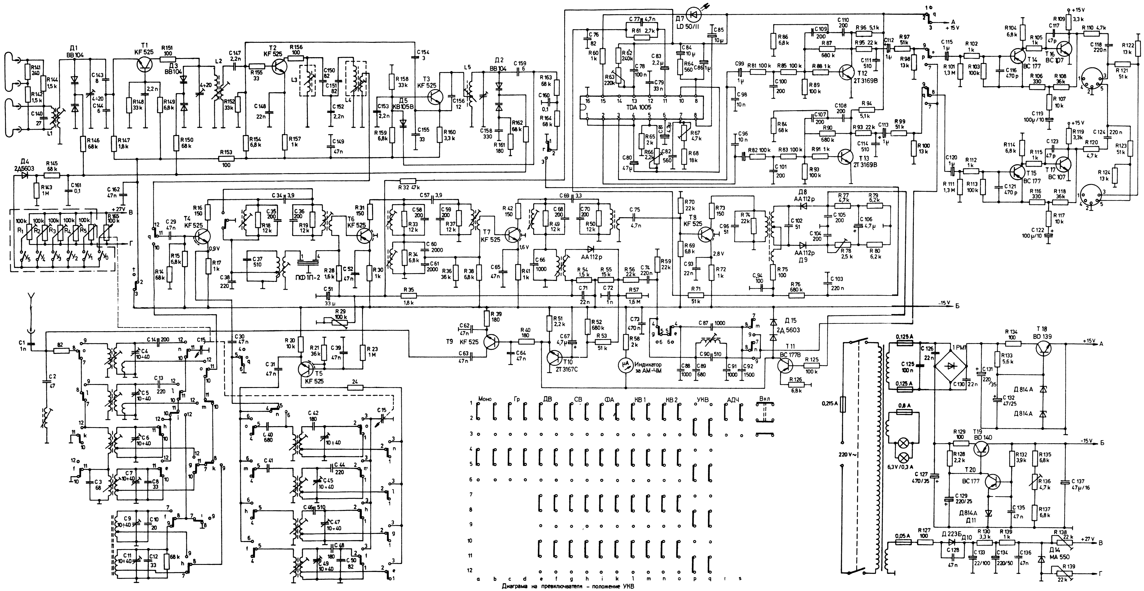
Диаграма на превключателя - положение УНВ
