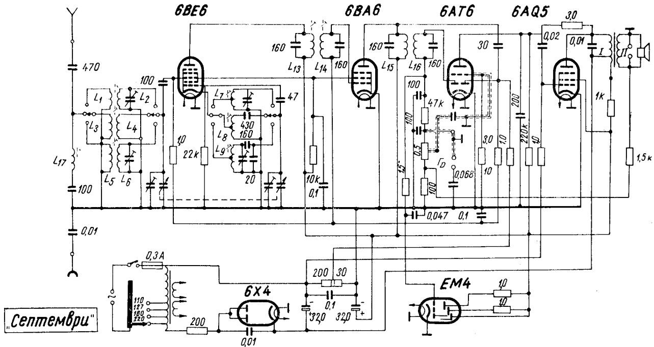
Фиг. 2.4.8. Схема на радиоприемника „Септември“ с лампи от миниатюрната серия
