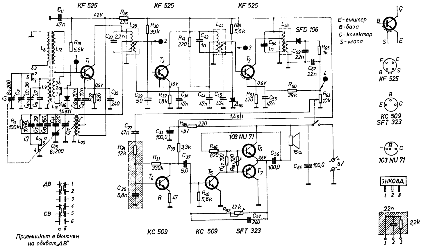
Фиг. 4.133. Принцилна схема на радиоприемник „Соло“
