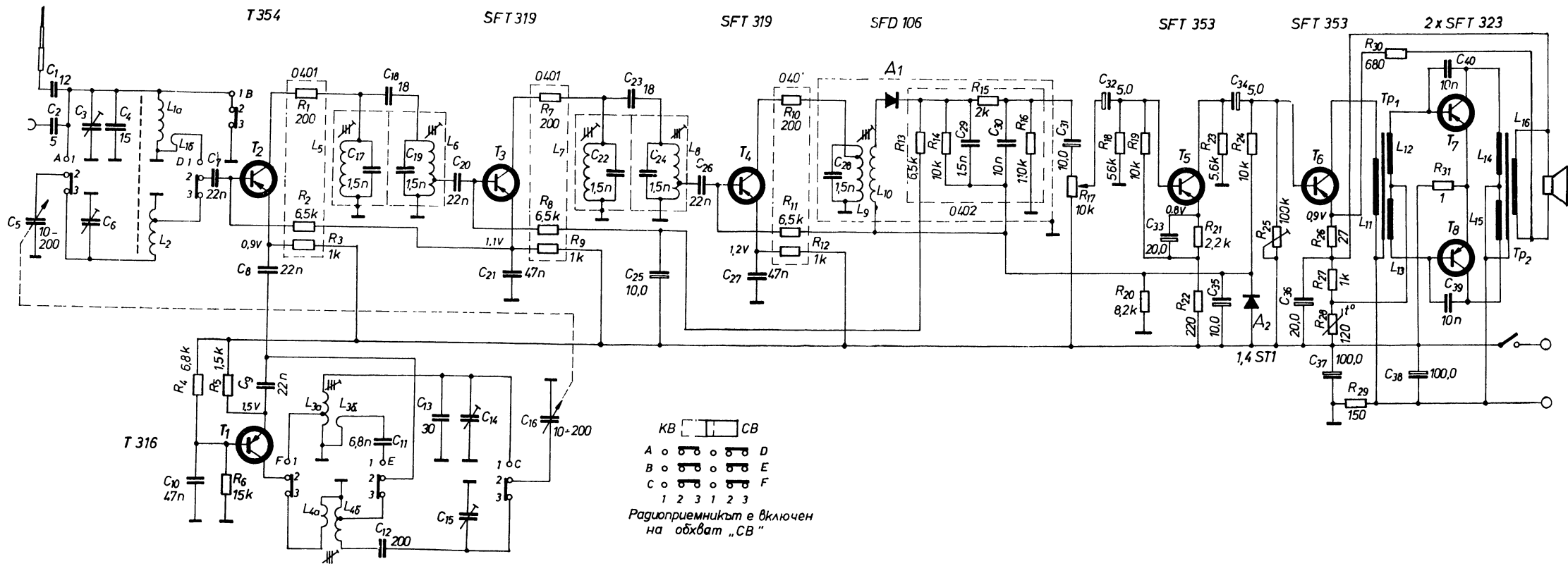
Фиг. 4.49. Принцилна схема на радиоприемник „Тенор“
