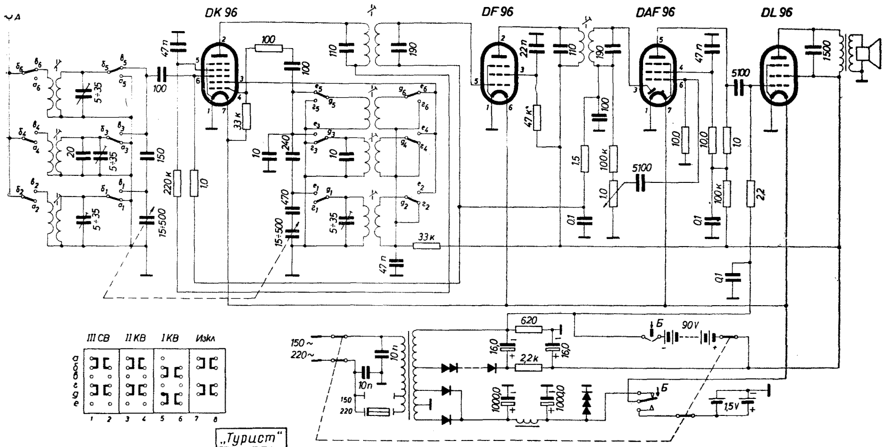
Фиг. 2.10.2. Схема на радиоприемника „Турист“
