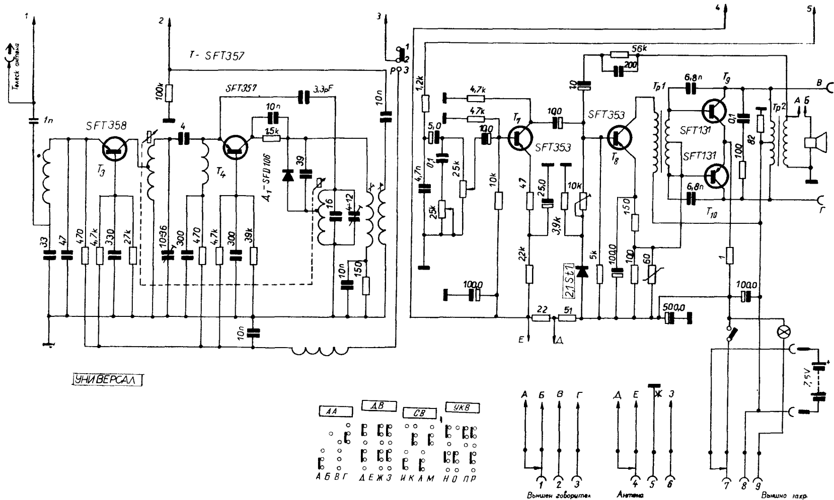
Фиг. 3.8.9. Схема на радиоприемника „Универсал“ (II част)
