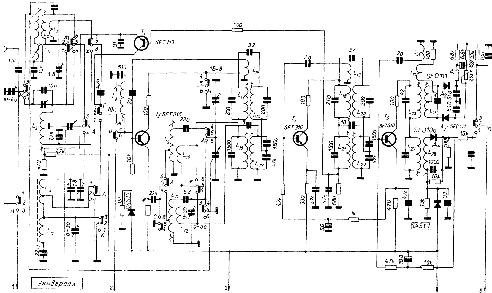
Фиг. 3.8.9. Схема на радиоприемника „Универсал“ (I част)
