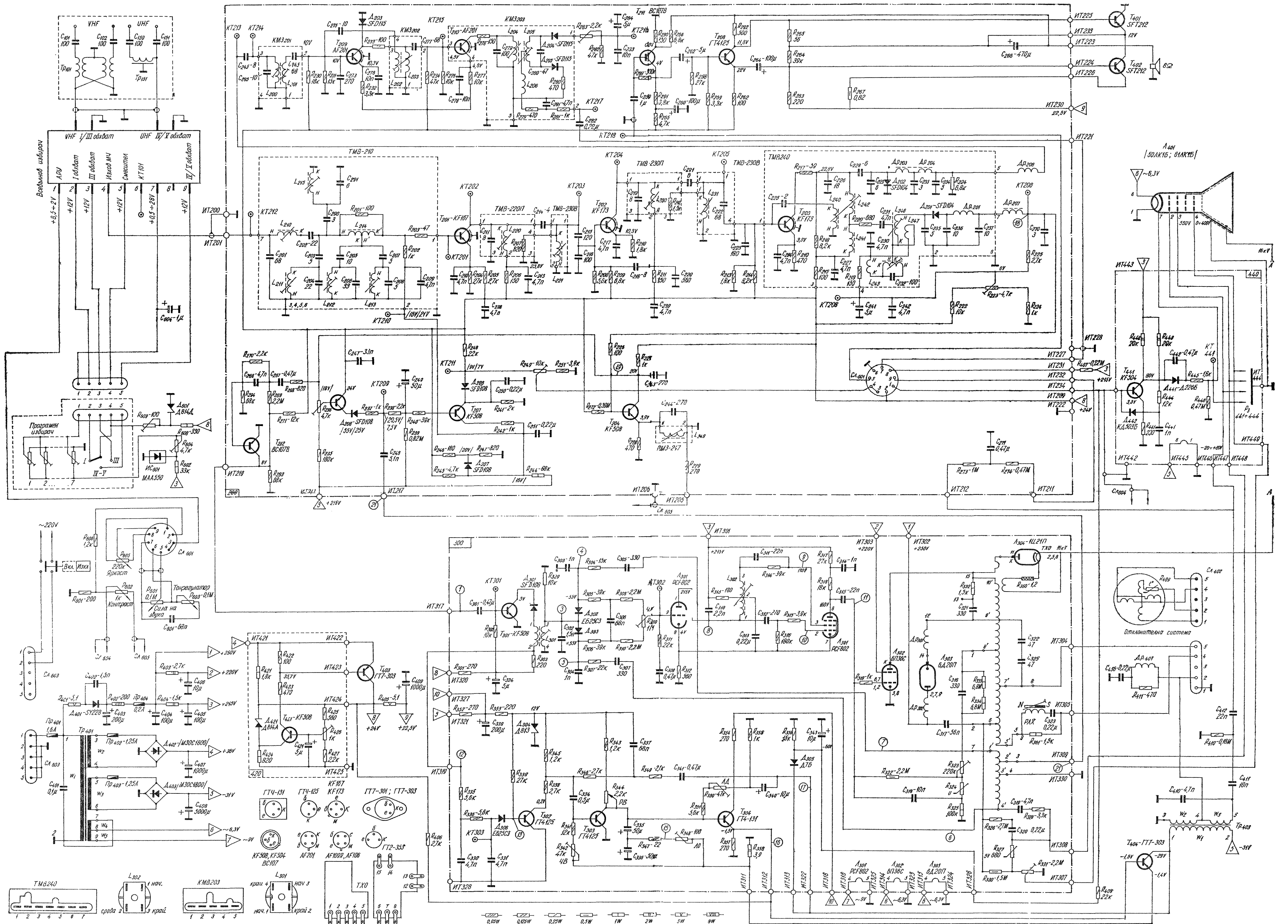
Приложение 4: Схема на телевизионен приемник „Содия 11“
