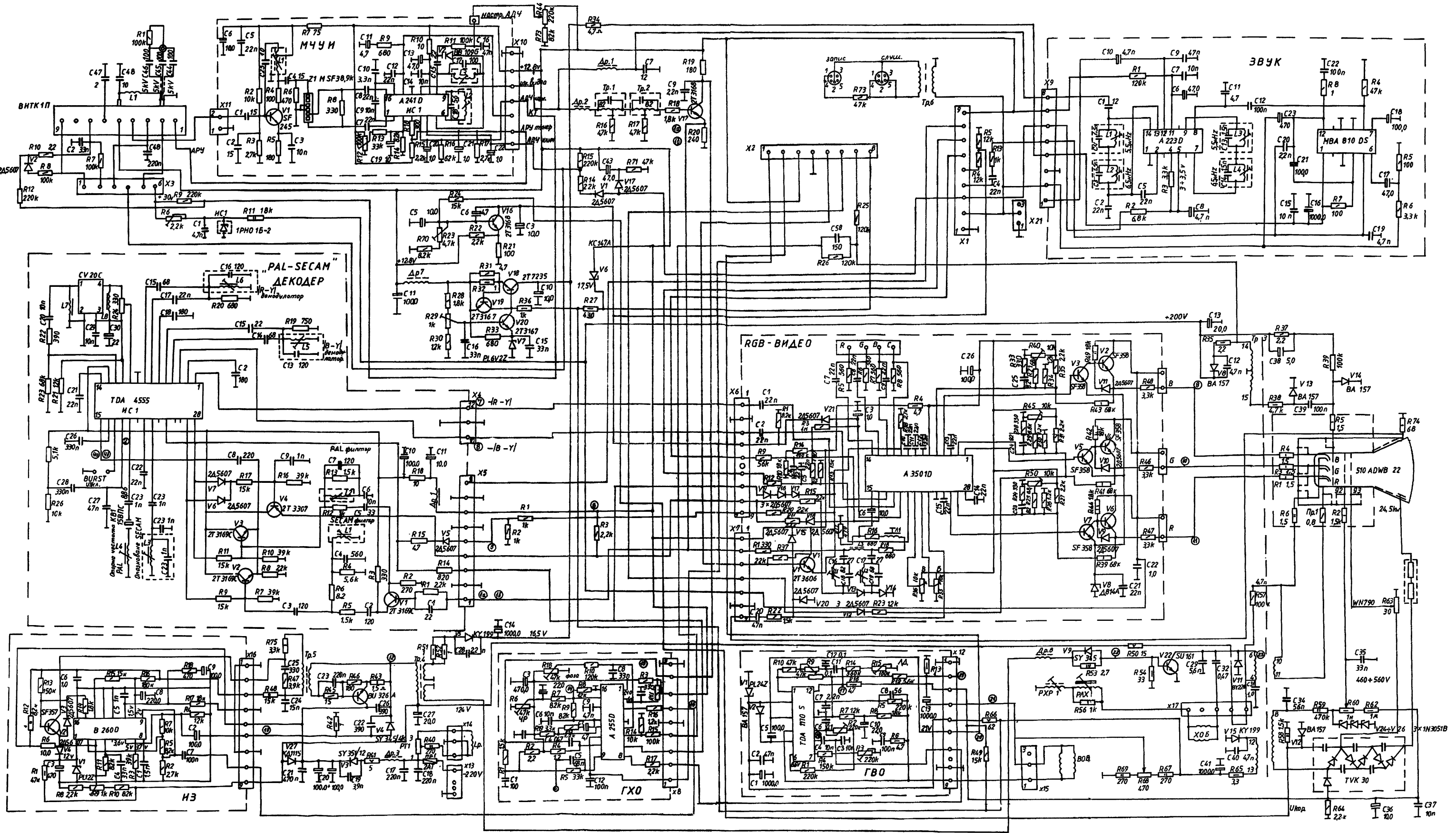
Ел.схема на "Велико Търново 882"-ТЦ 5103
