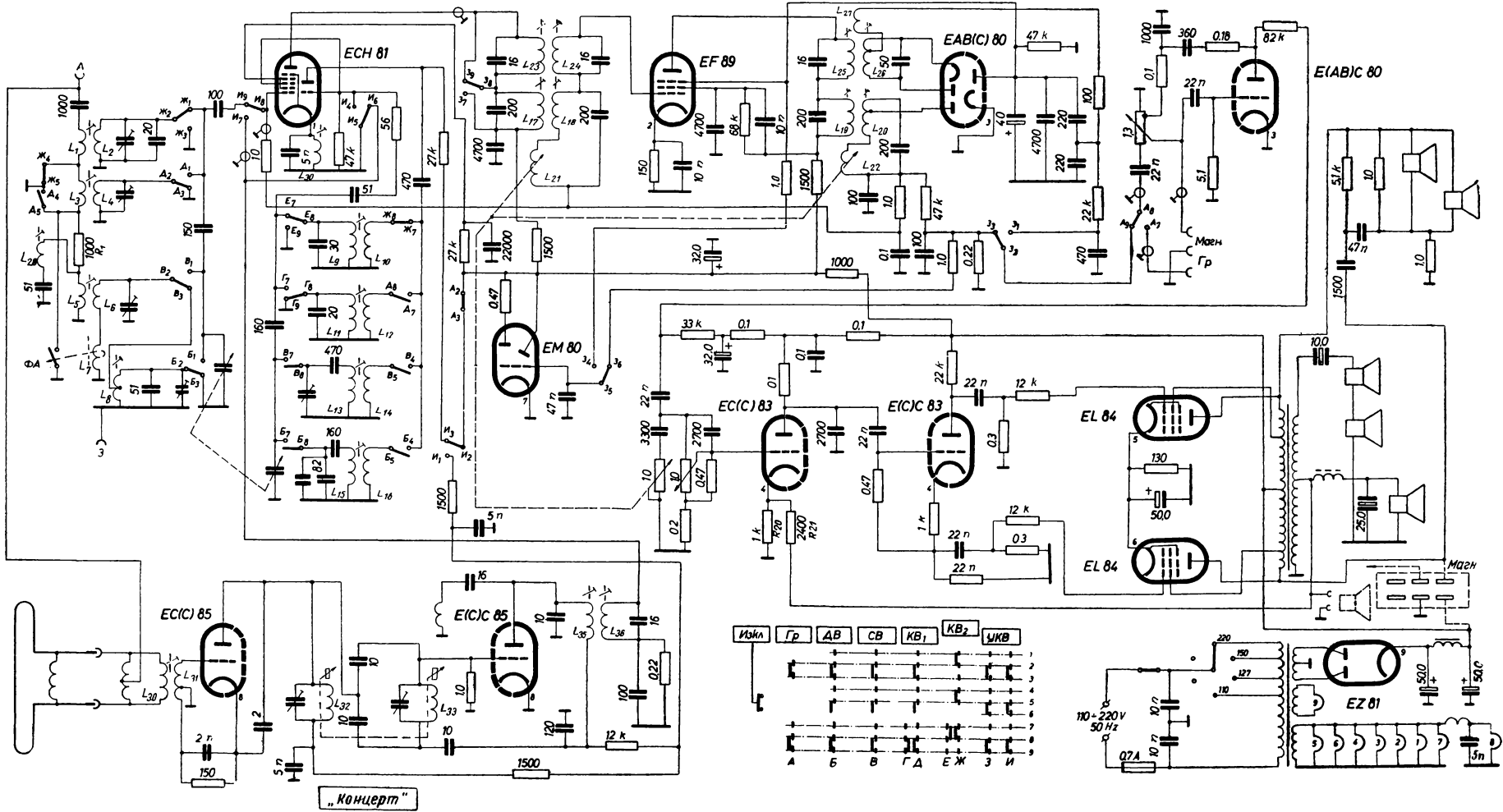
Фиг. 2.13.4. Схема на радиоприемника „Концерт“
