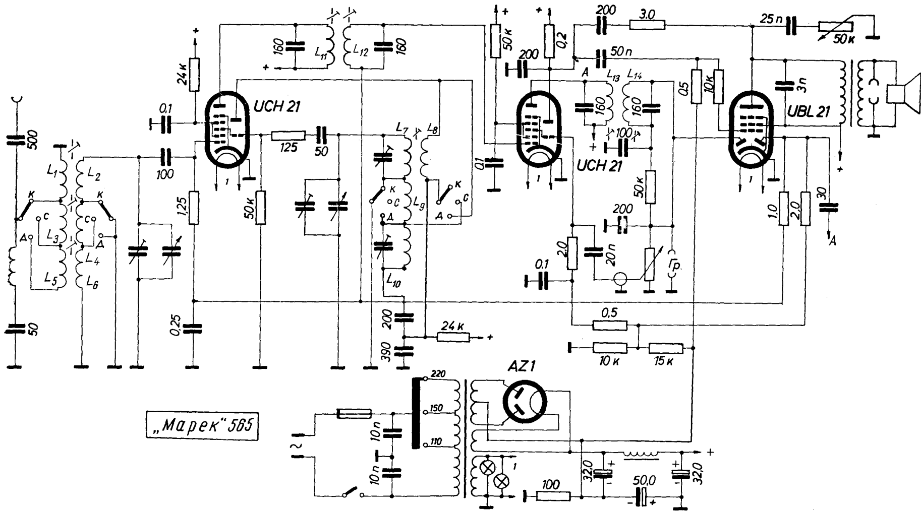
Фиг. 2.5.6. Схема на радиоприемника „Марек“ 565 с лампи серия U
