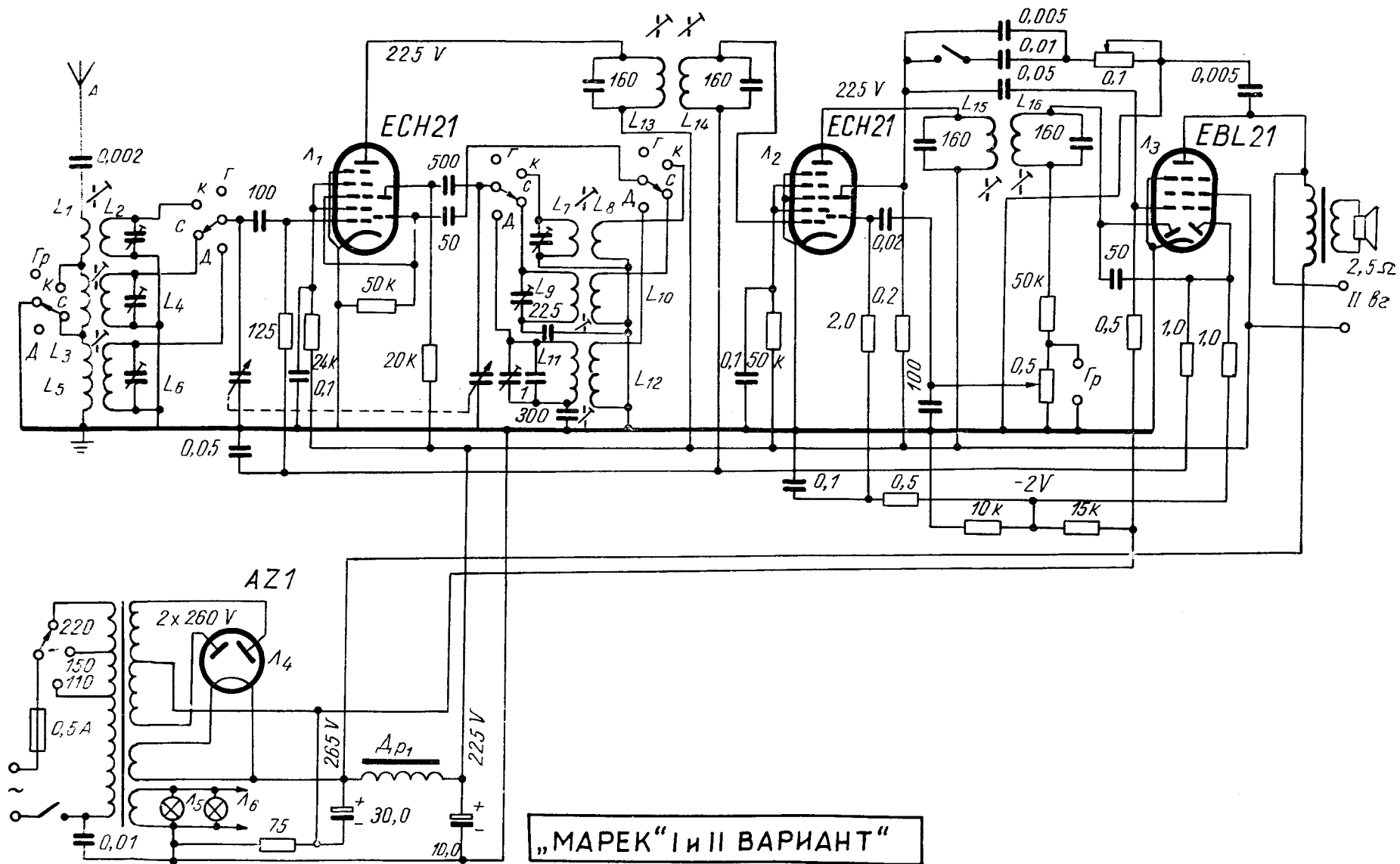
Фиг. 2.5.3. Схема на радиоприемника „Марек“ I и II вариант
