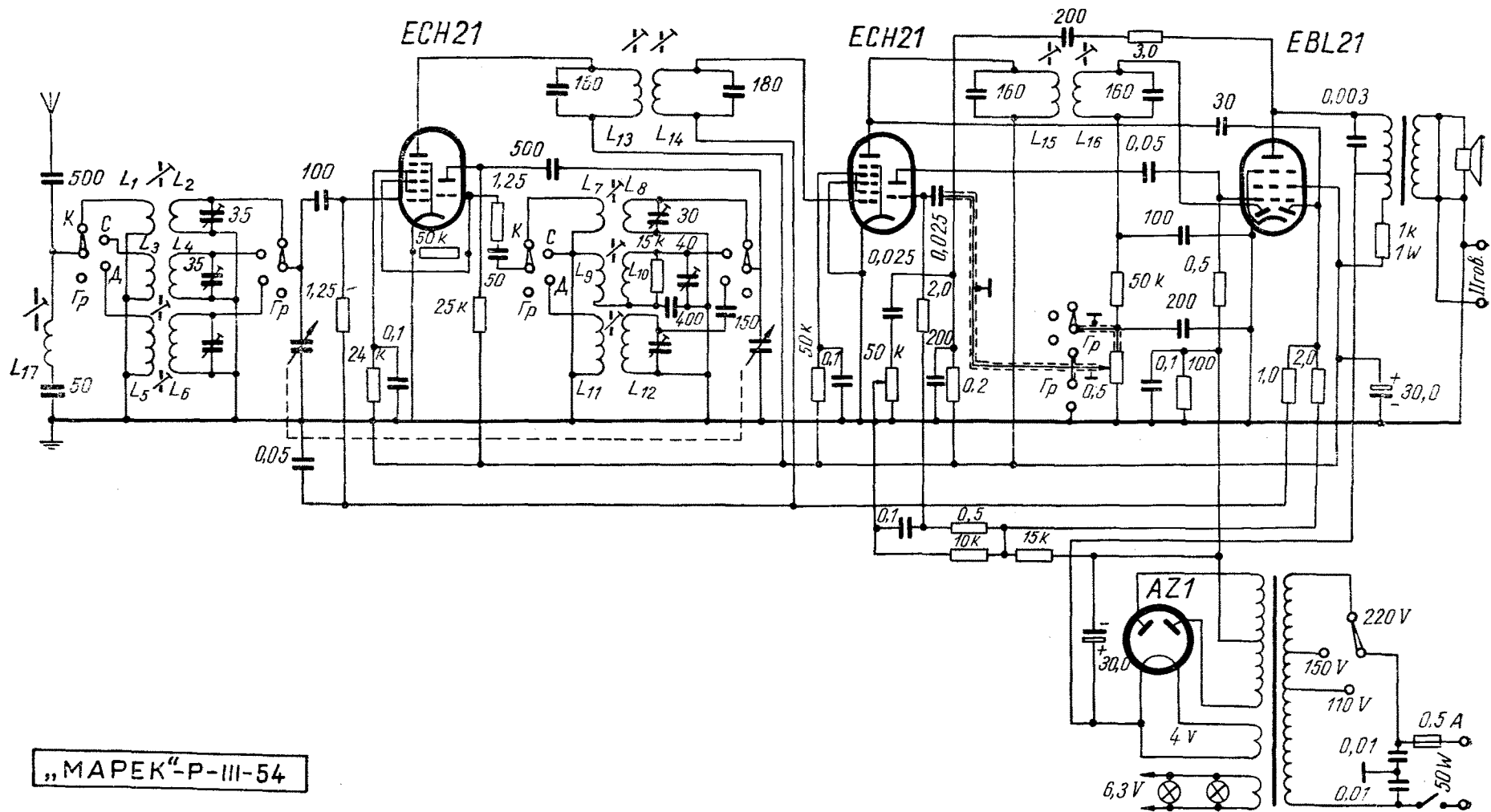
Фиг. 2.5.4. Схема на радиоприемника „Марек“ P-III-54
