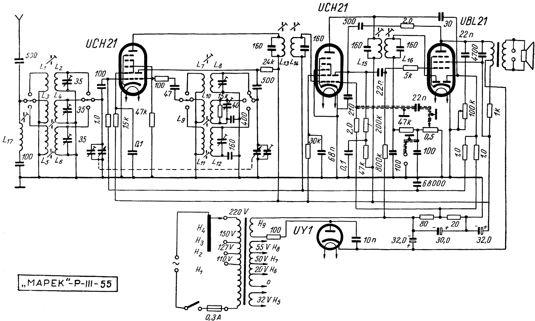
Фиг. 2.5.5. Схема на радиоприемника „Марек“ Р-III-55 с лампи серия U.
