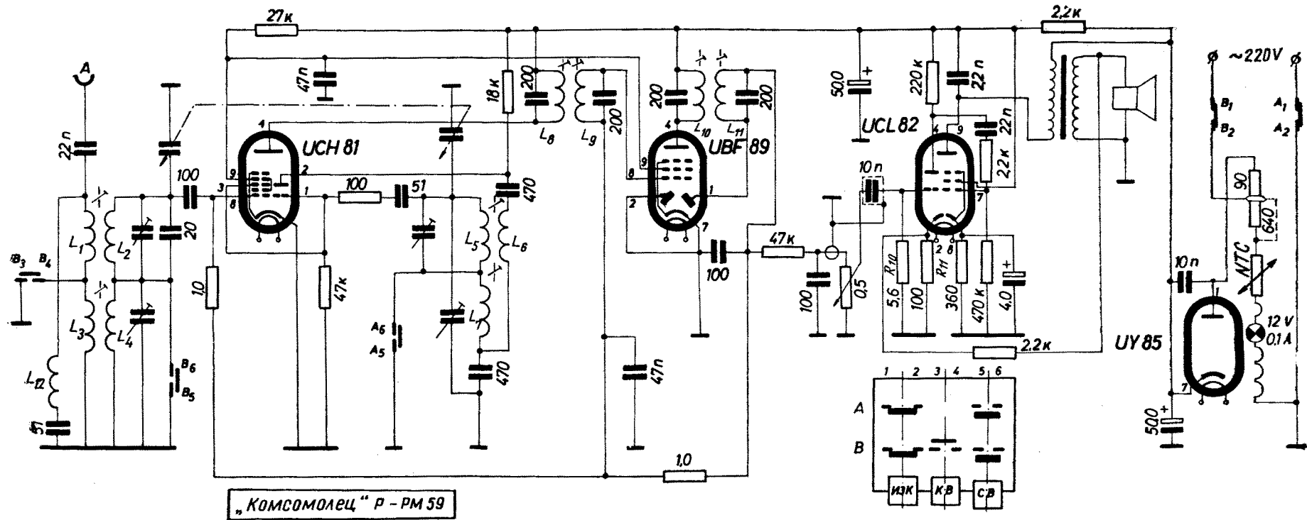
Фиг. 2.12.3. Схема на радиоприемника „Комсомолец“
