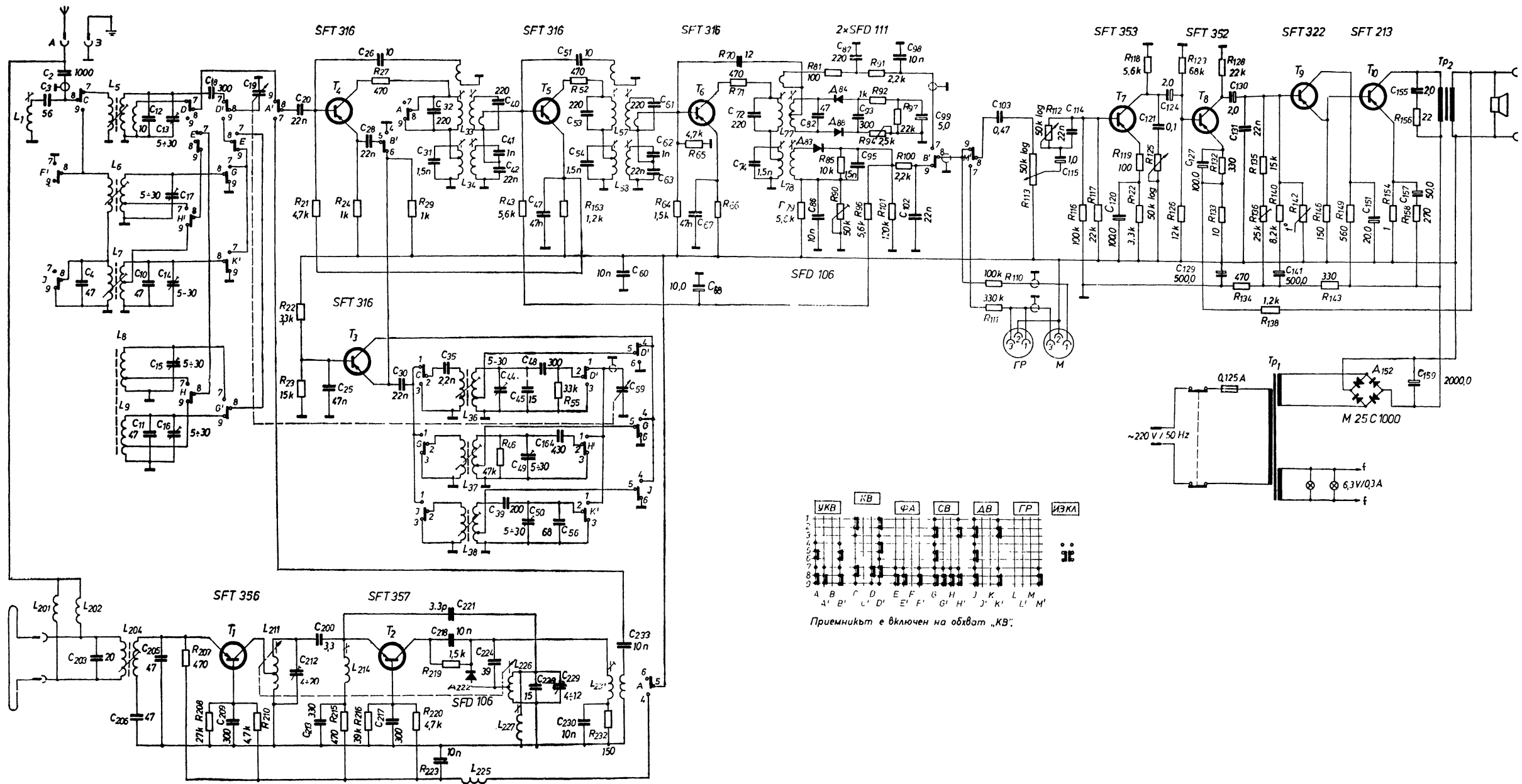
Фиг. 4.71. Приципна схема на радиоприемник „Рила“
