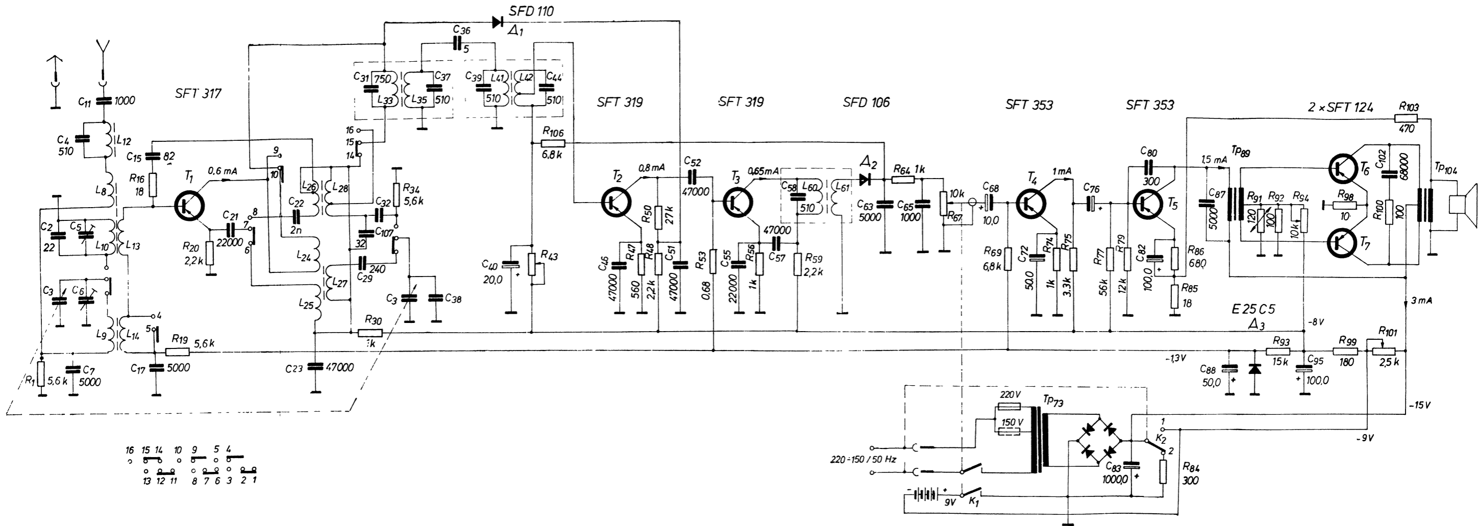
Фиг. 4.40. Принципна схема на радиоприемник „РМС 10-Т“
