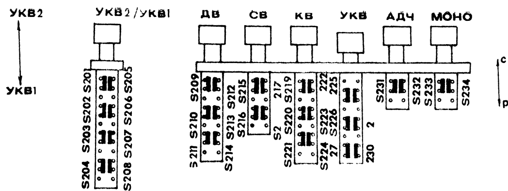
БУТОНЕН ПРЕВКЛЮЧВАТЕЛ В4 ЧАСТ ВКЛЮЧЕН ОБХВАТ УКВ
